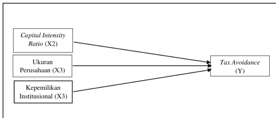
Gambar 1. Desain Penelitian
